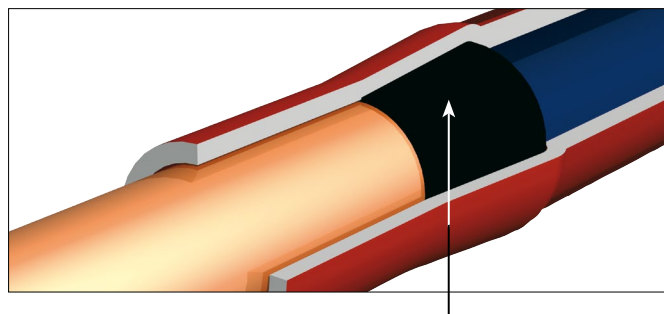
Einfaches Aufziehen auf Rohrleitungen durch Gleitfolie
