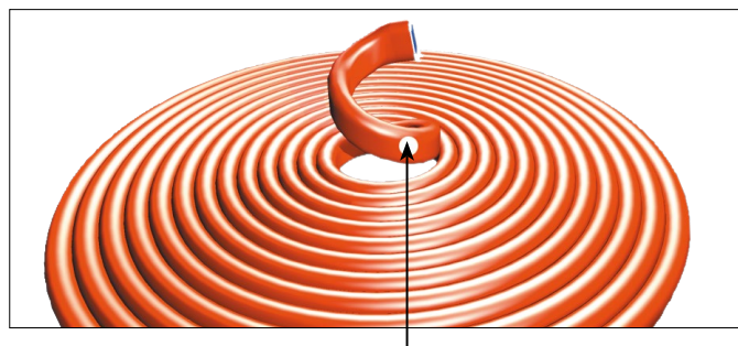
Klebepunkte im Abstand von ca. 1 m verhindern das Auseinanderfallen der Rolle
